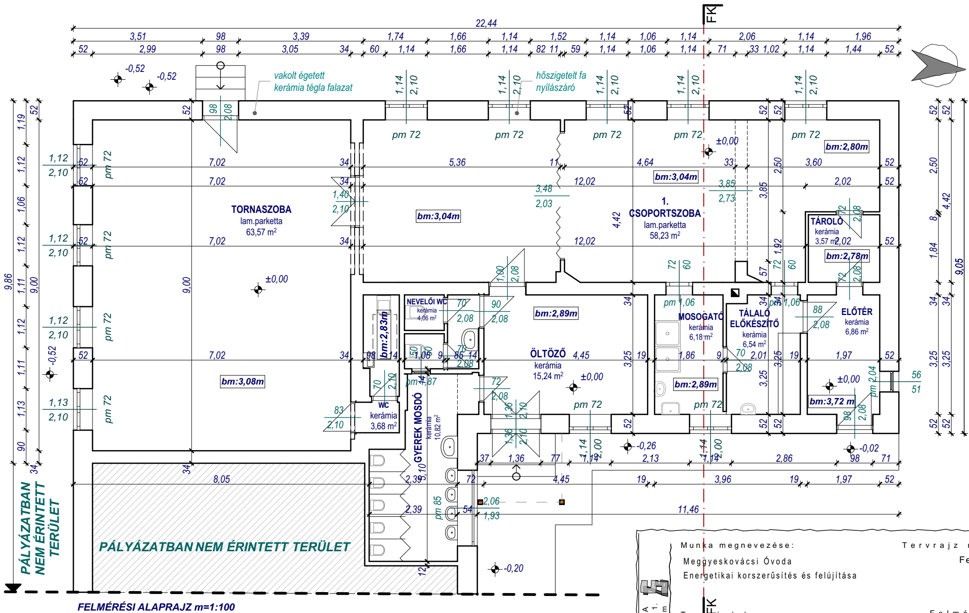
FELMÉRÉSI ALAPRAJZ m=1:100
