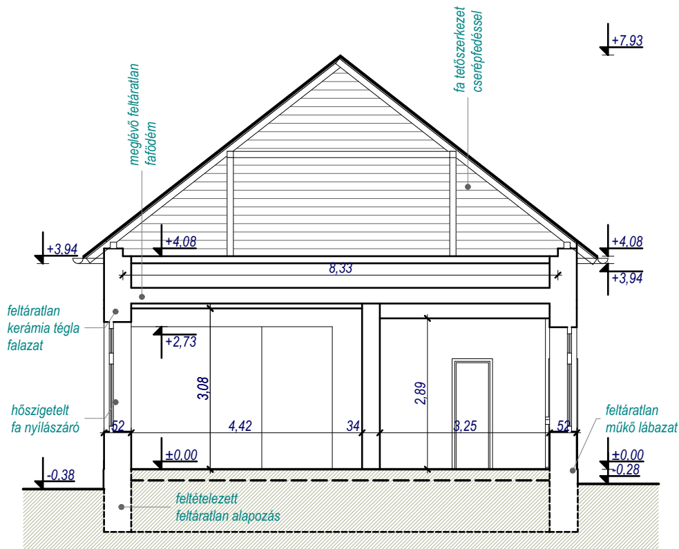
Keresztmetszet m=1:100
